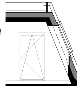
SCHNITT 1-1
