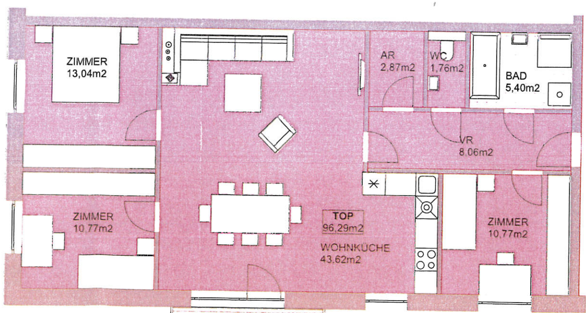
WOHNUNG M 1:100
