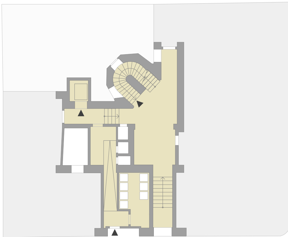
GRUNDRISS EG
