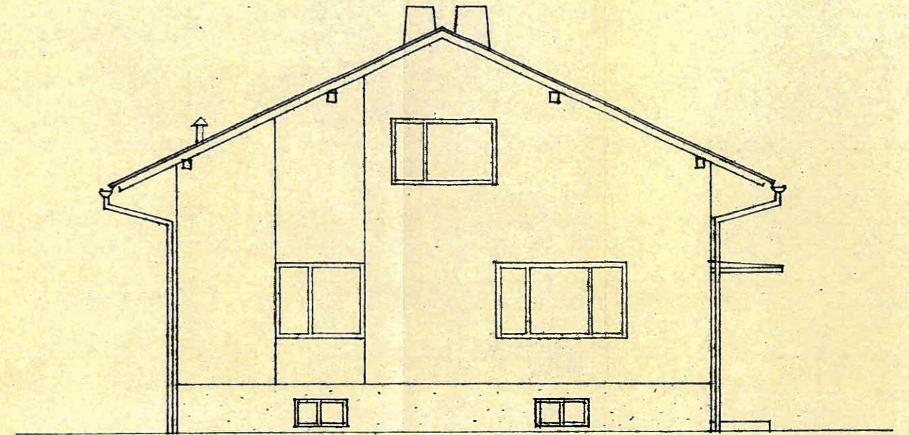
SÜDWESTANSICHT
