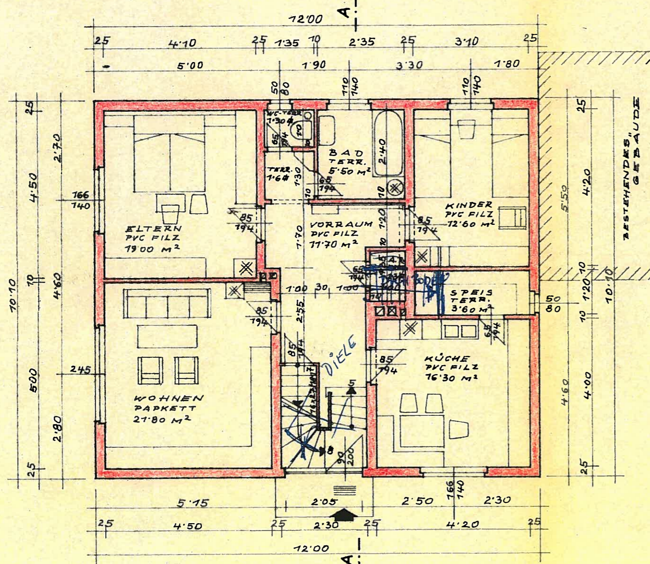
ERDGESCHOSS
