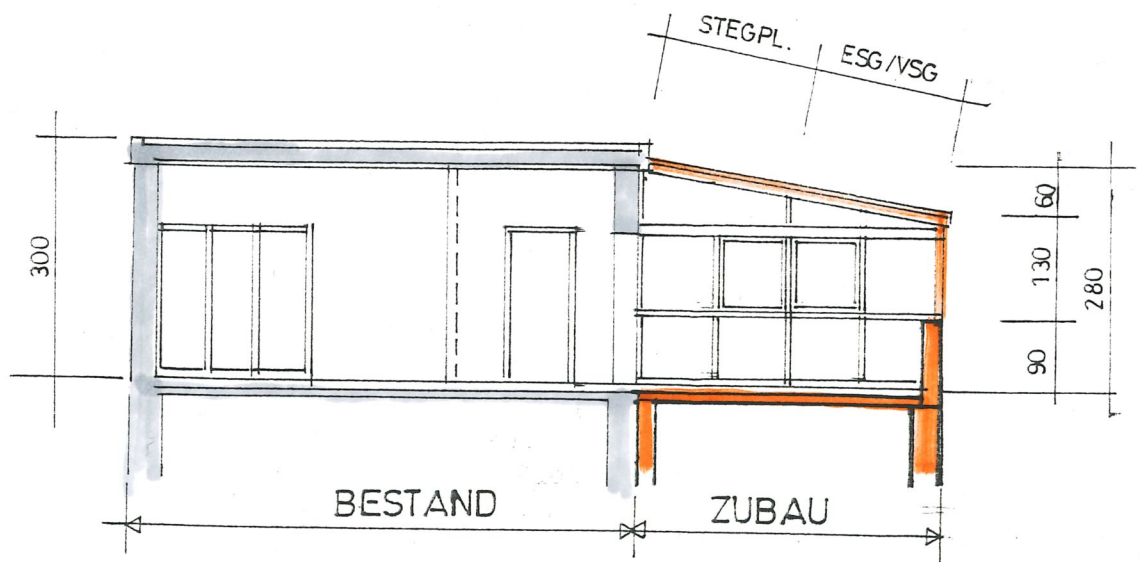
SCHNITT 1 - 1
