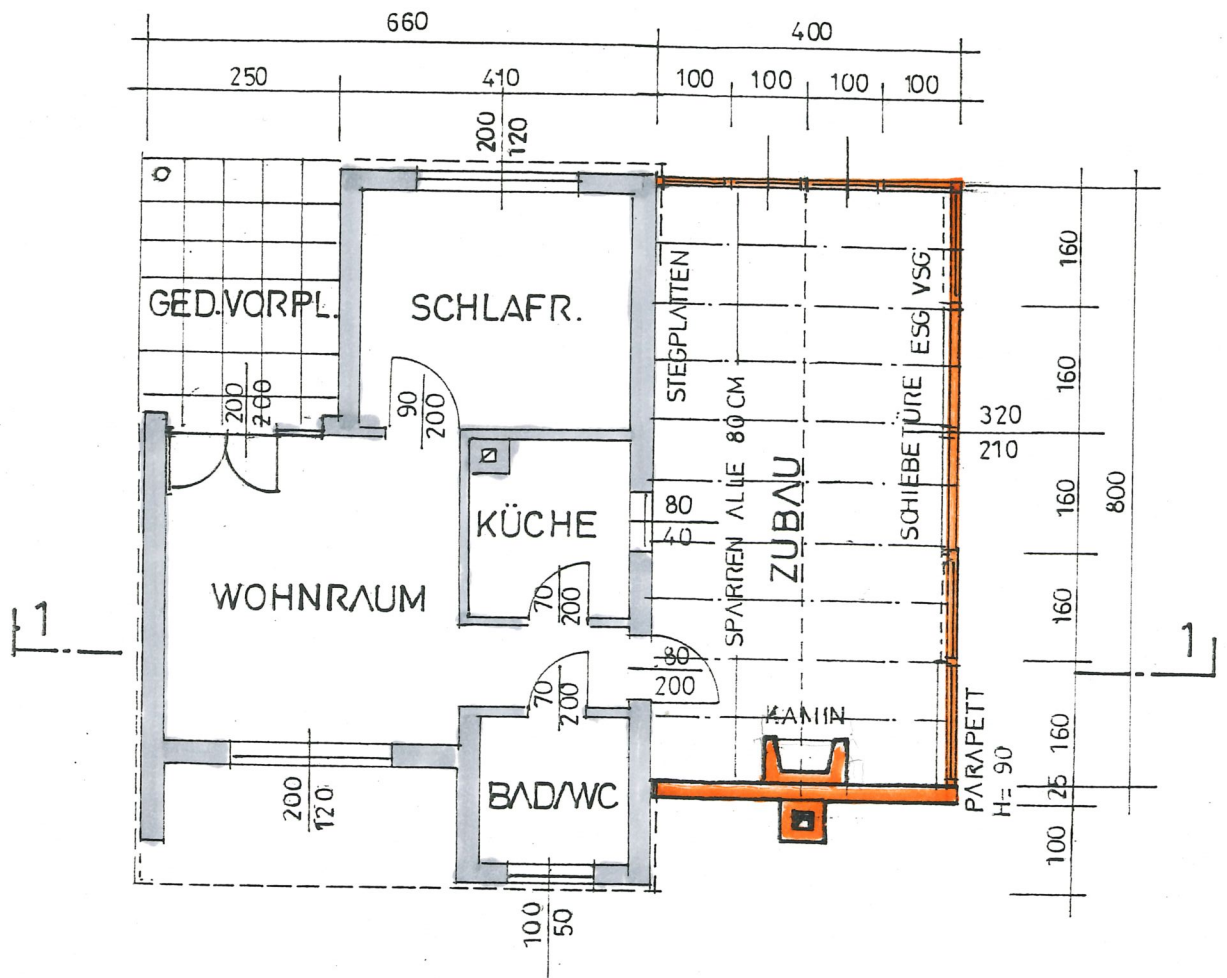
GRUNDRISS
