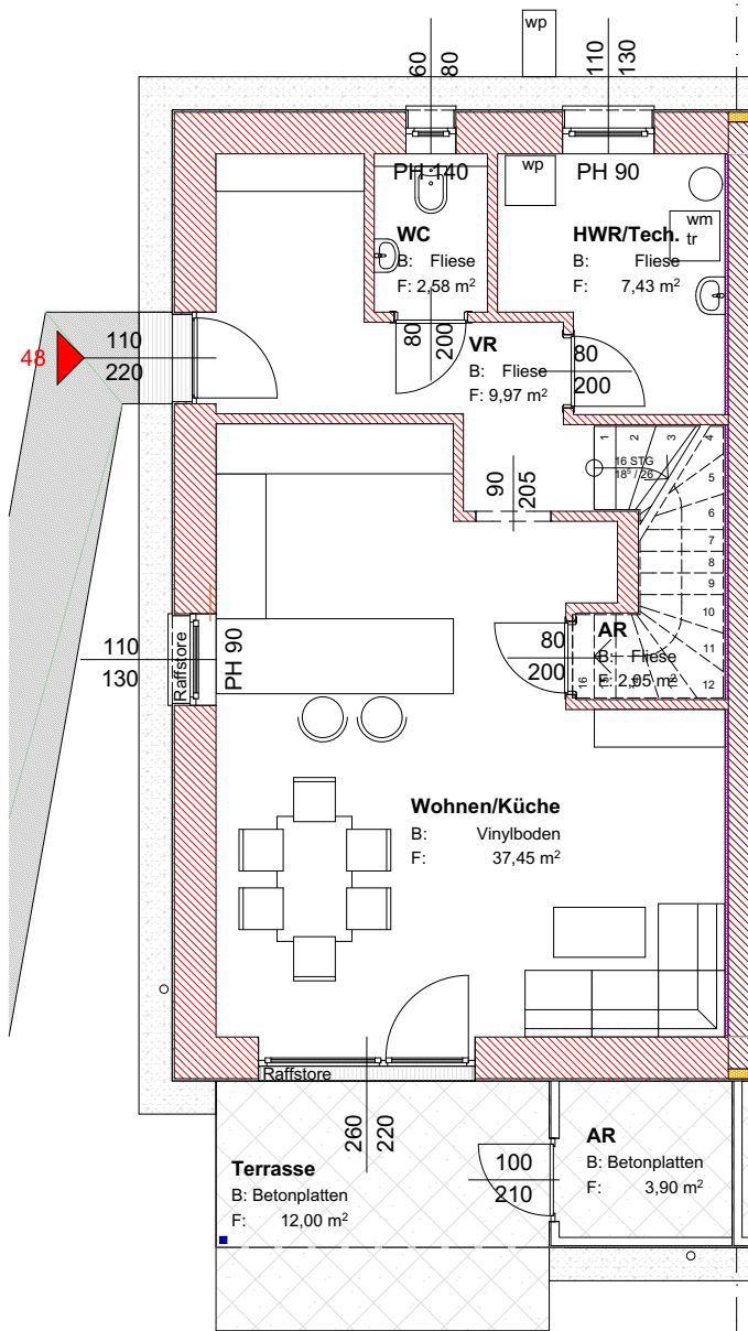
0. Erdgeschoss 1:100
