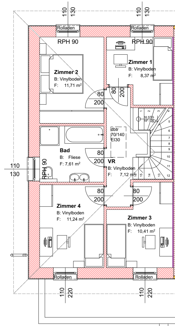
1. Obergeschoss 1:100
