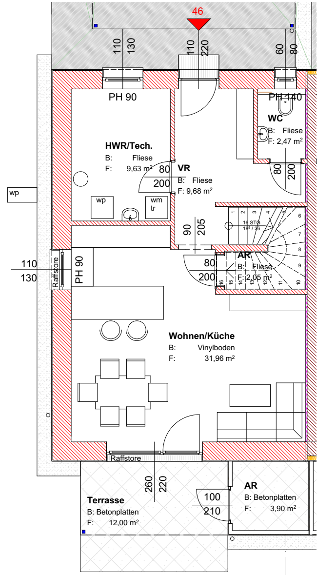
0. Erdgeschoss 1:100
