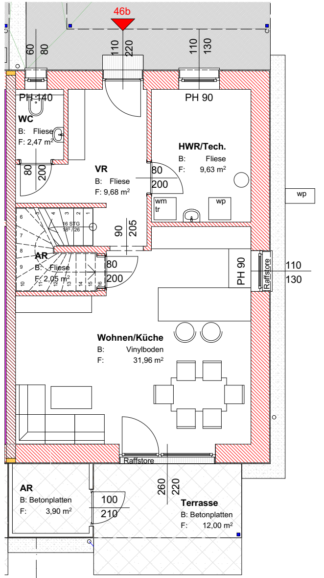
0. Erdgeschoss 1:100
