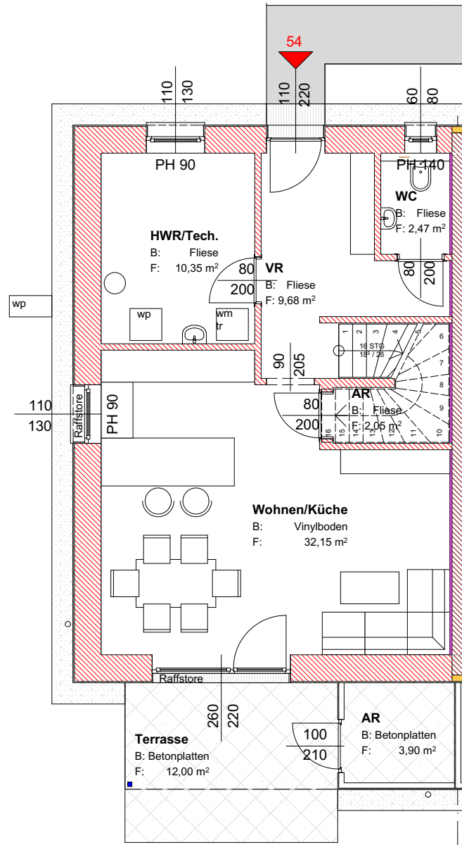
0. Erdgeschoss 1:100
