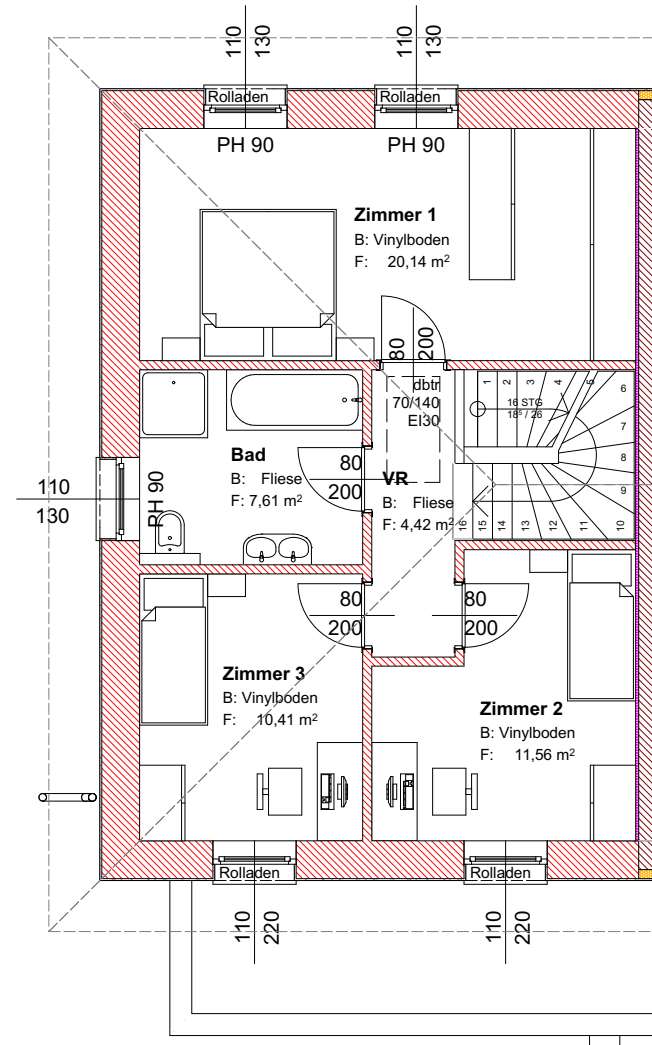
1. Obergeschoss 1:100
