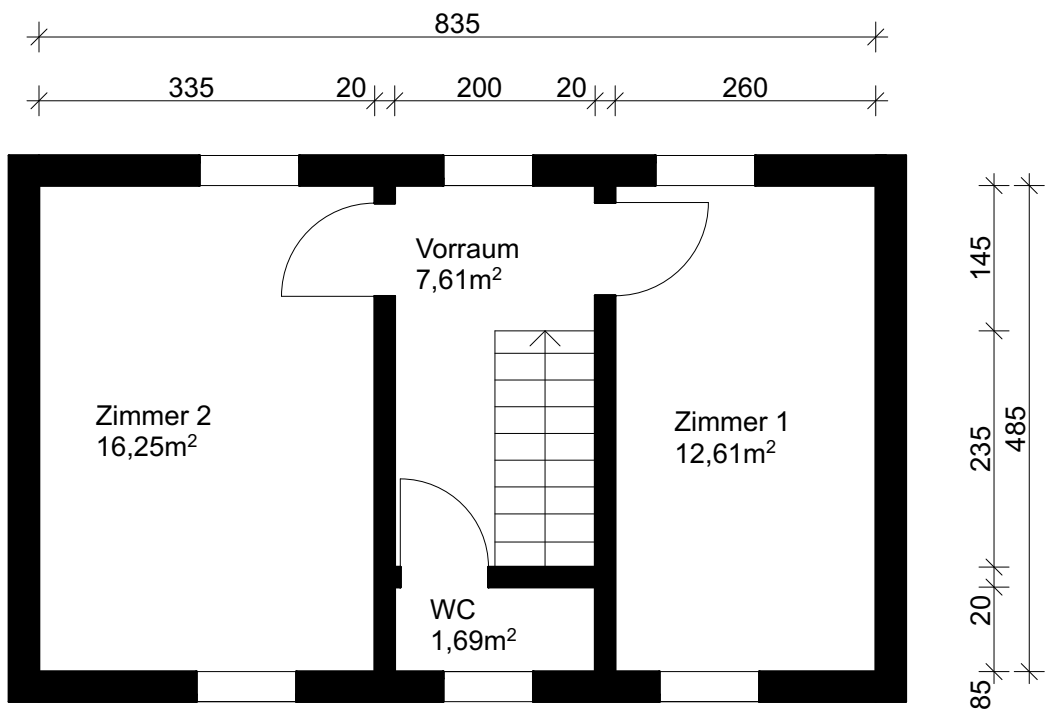
Obergeschoss
