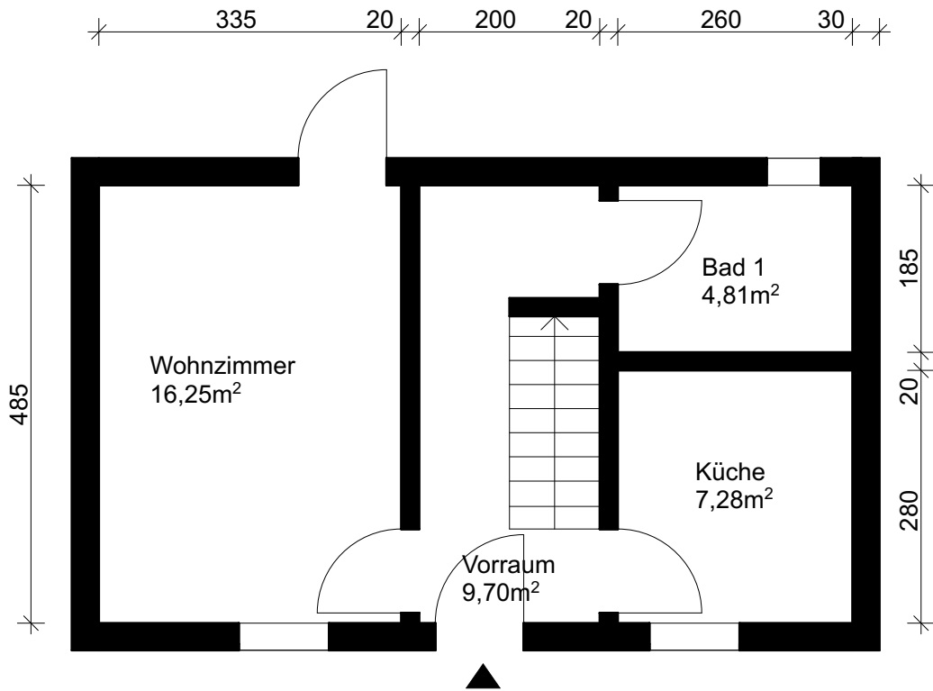
Erdgeschoss
