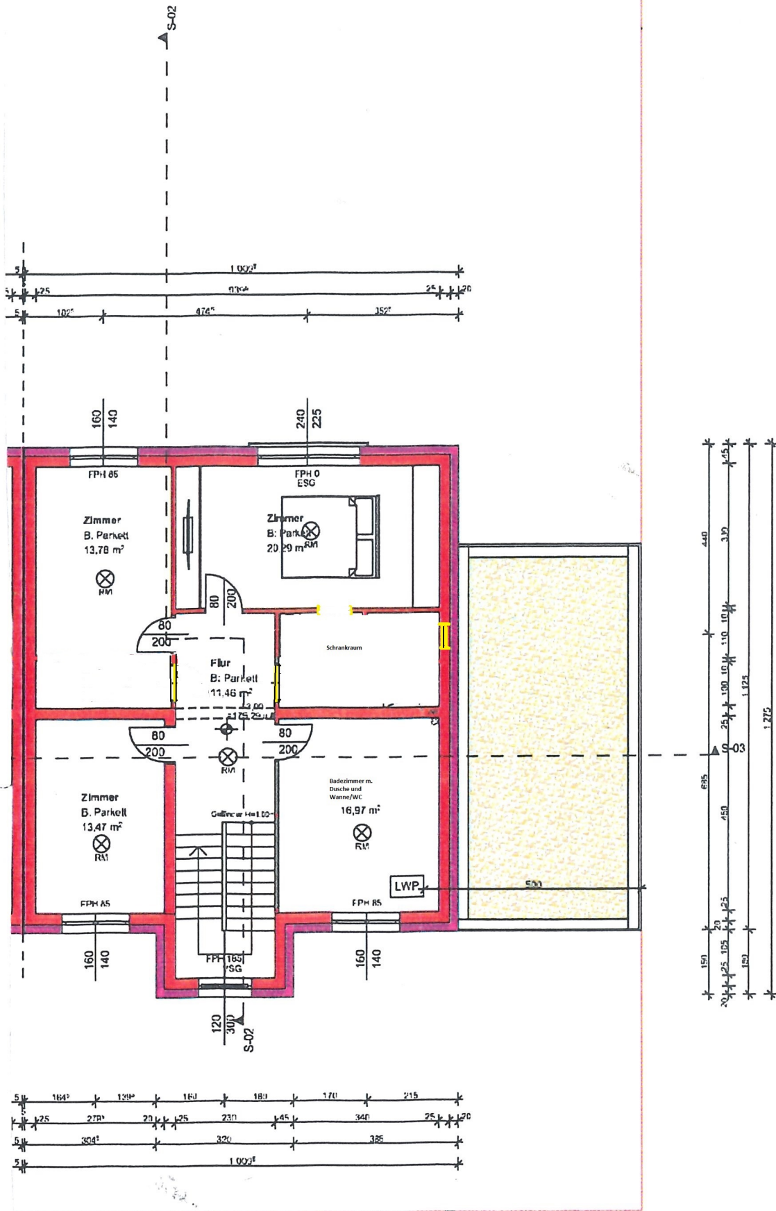
Grundriss OG WNF:87,75 m 2 M 1:100
