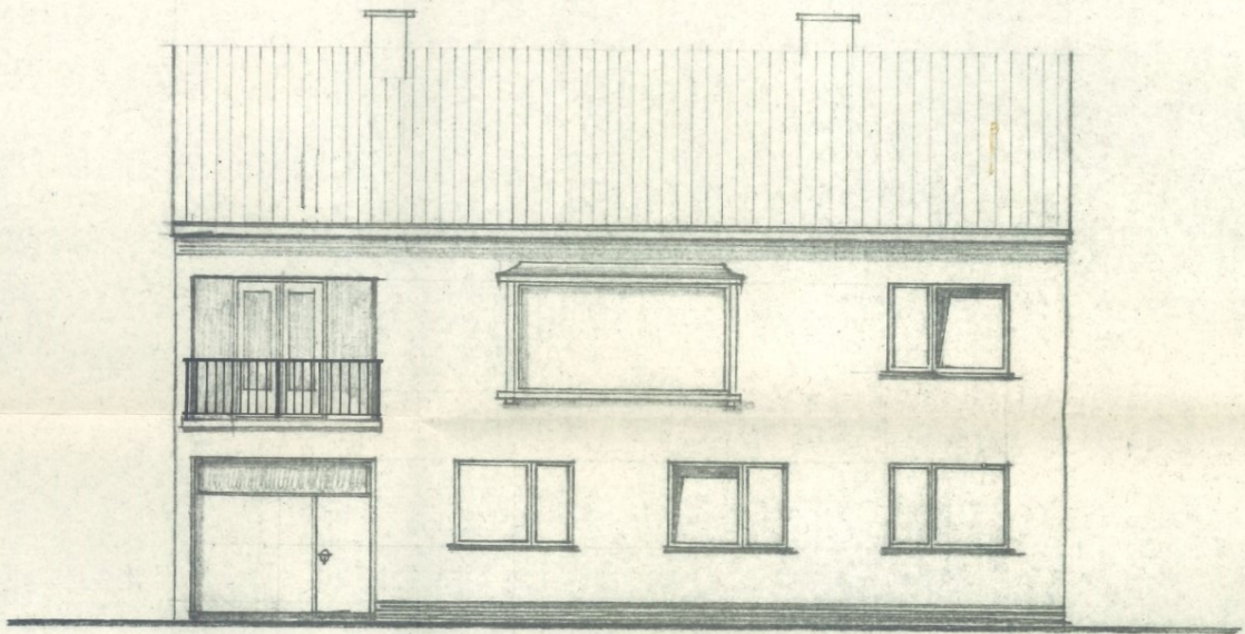
STRASSENANSICHT:
