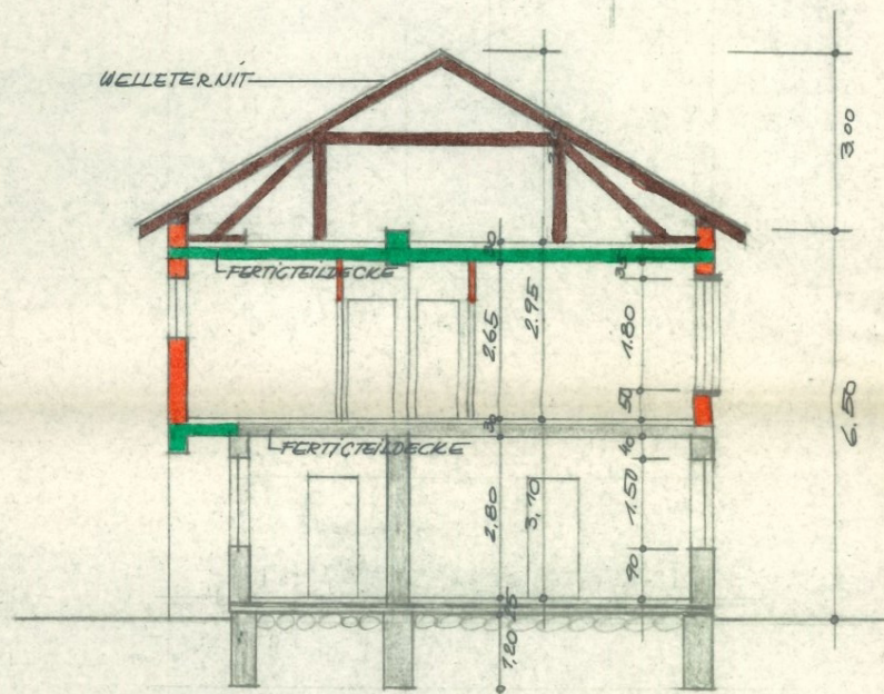
SCHNITT A-B
