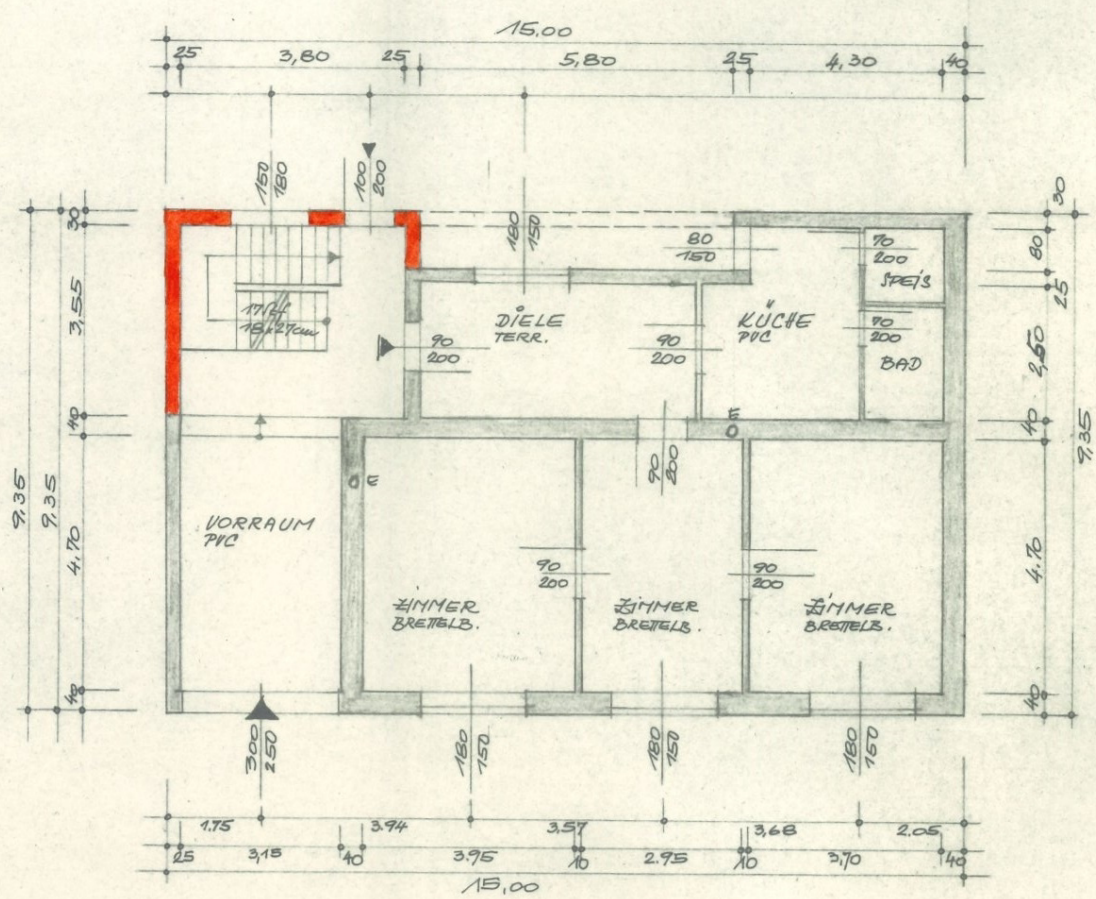
ERDGESCHOSS:
