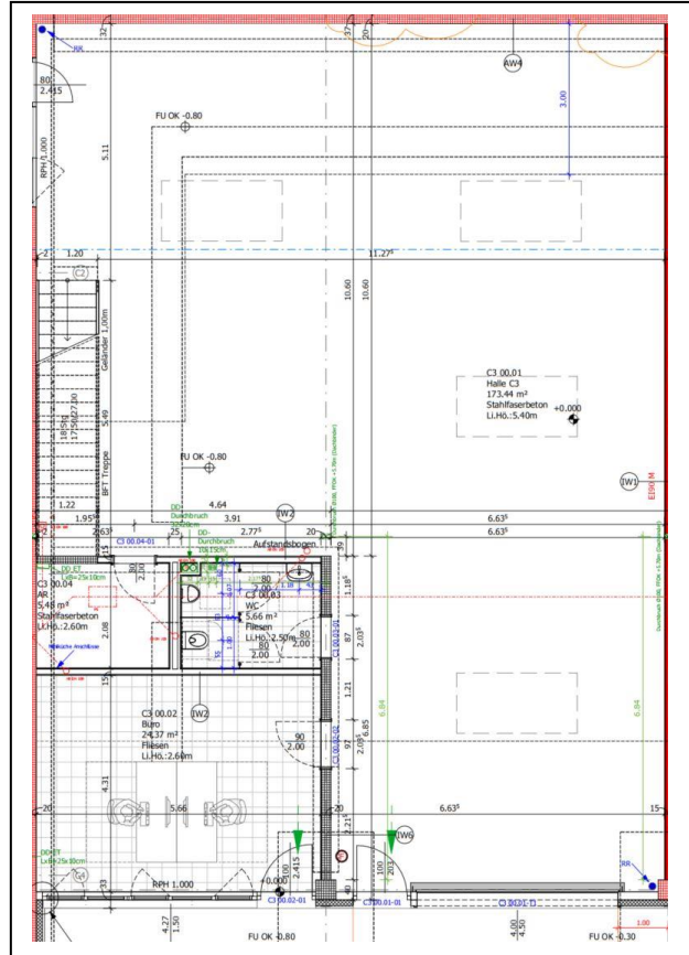
Erdgeschoss
