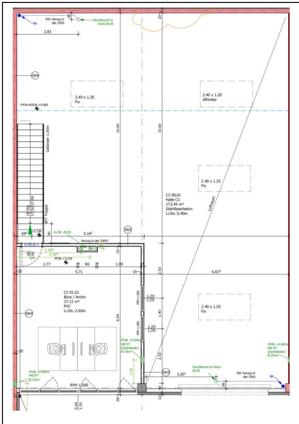
Obergeschoss
