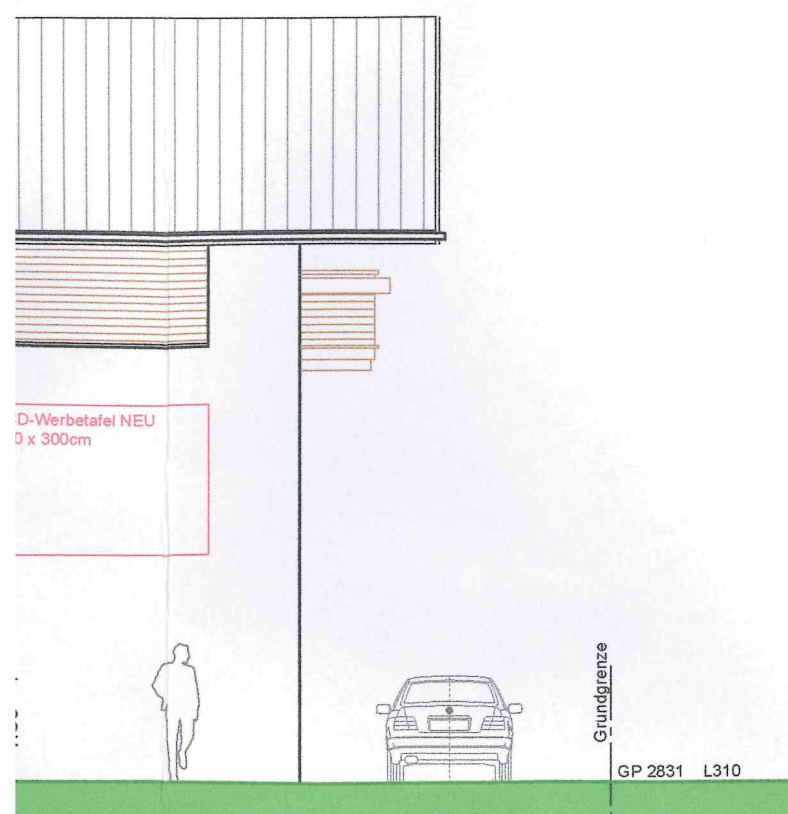
Schnitt A-A
