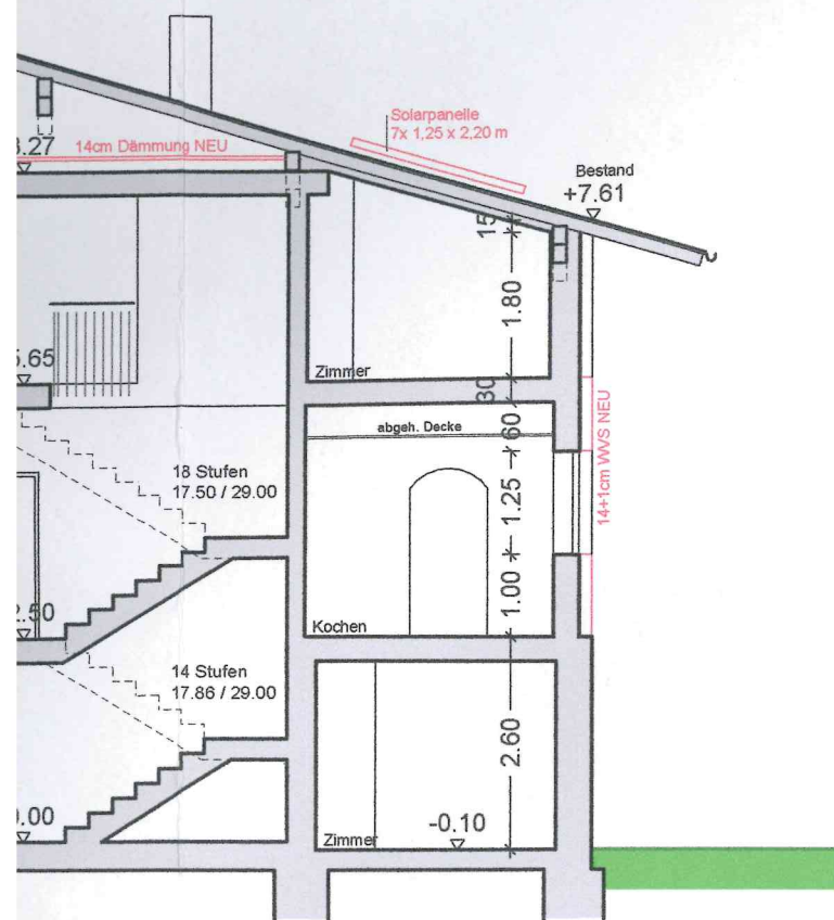
Schnitt A-A
