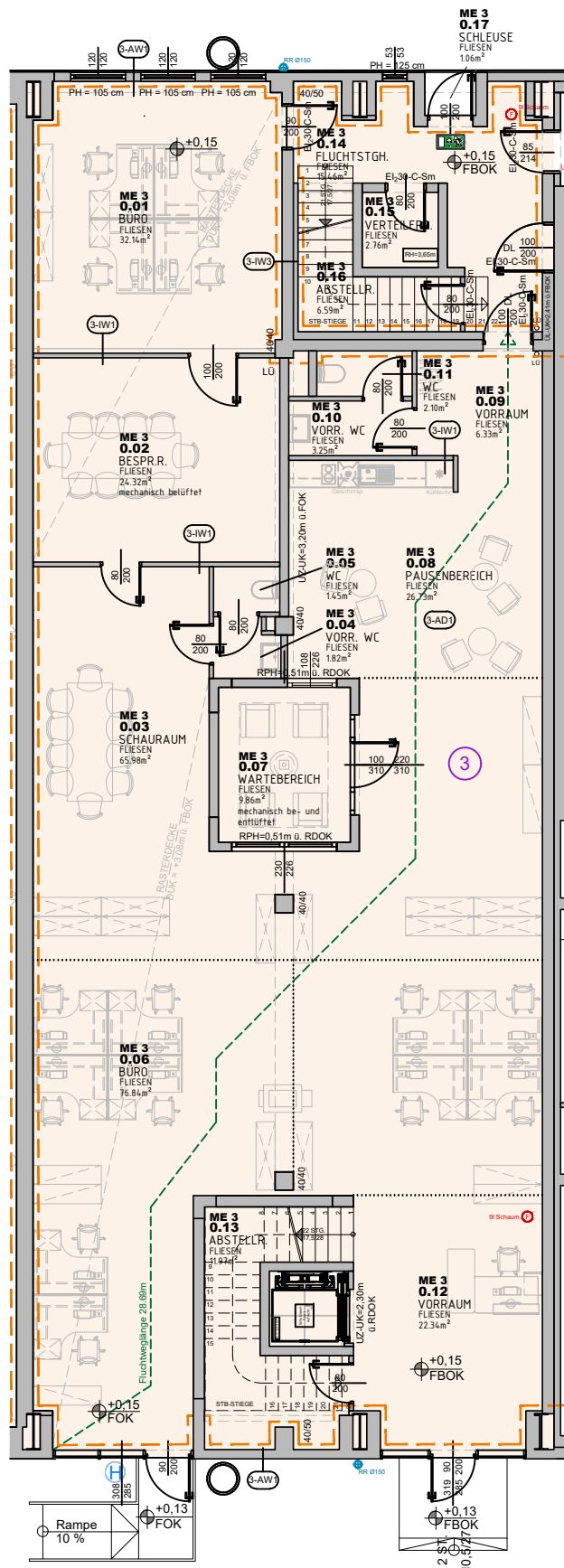
ERDGESCHOSS MIETEINHEIT 3 GESAMTFLÄCHE: 309,94m 2
