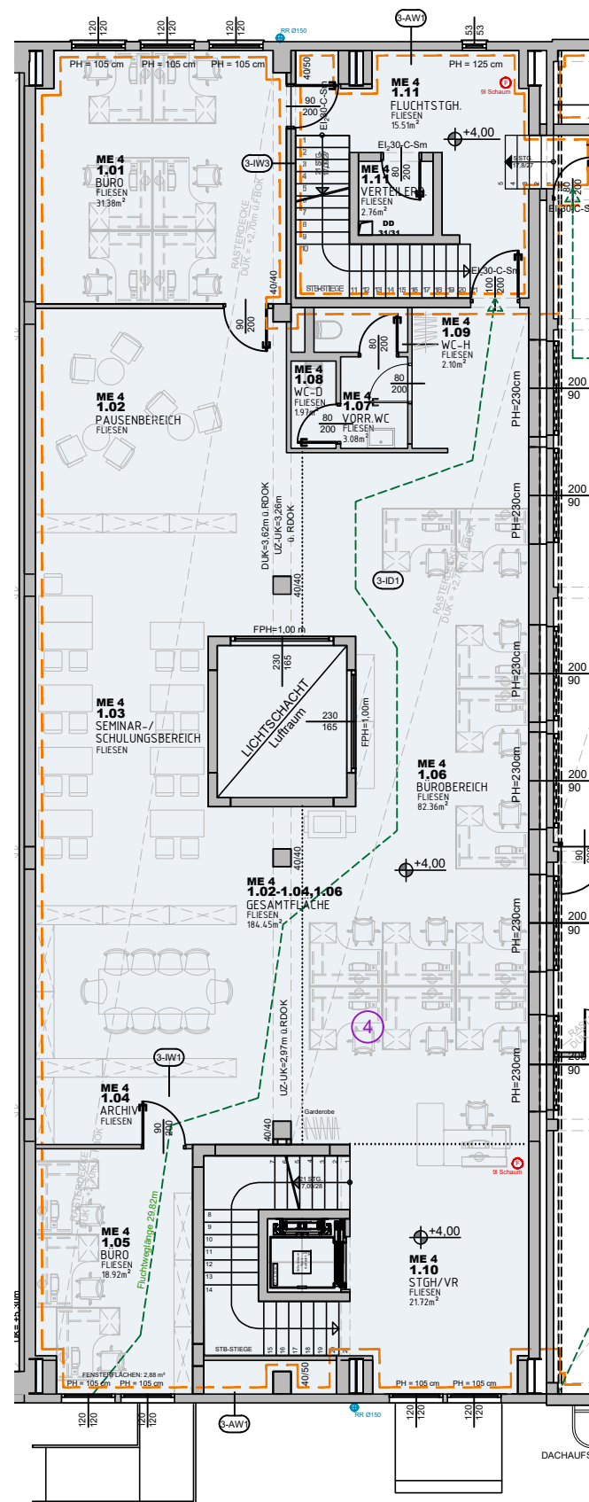
1. OBERGESCHOSS MIETEINHEIT 4 GESAMTFLÄCHE: 281,89m 2
