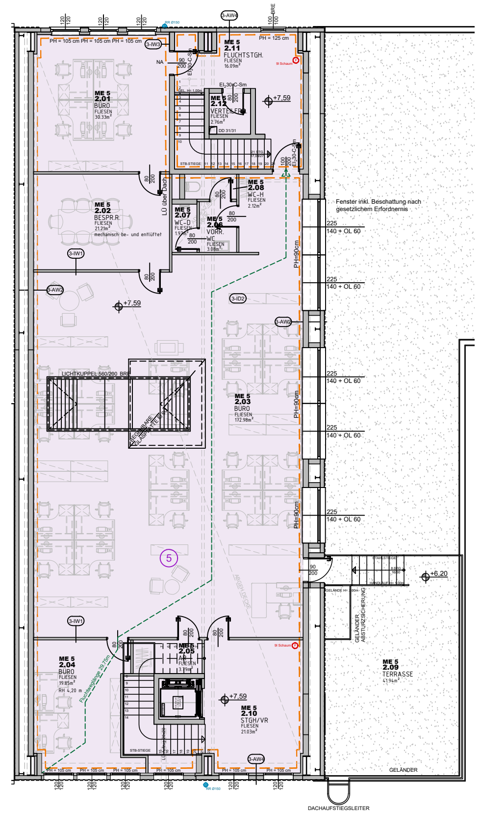
2. OBERGESCHOSS MIETEINHEIT 5 GESAMTFLÄCHE: 295,21m 2 (exkl. Terrasse 41,94m 2 )
