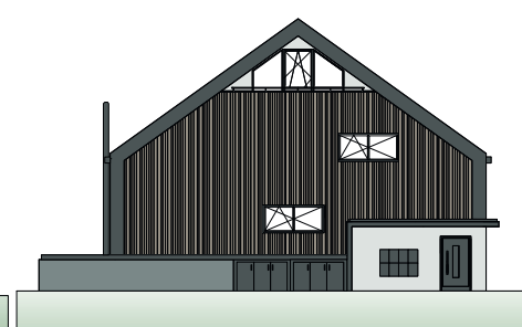
Ansicht Ost
