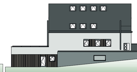
Ansicht Süd
