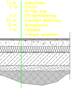
BODENAUFBAU M 1:10 Nassseinheiten, TR, Lager
