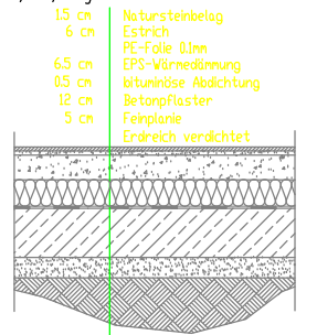
BODENAUFBAU M 1:10 Nassseinheiten, TR, Lager
