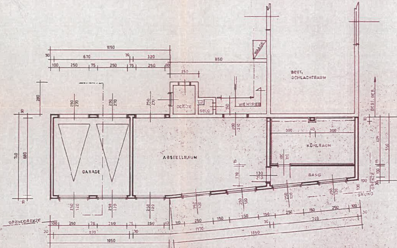
GRUNDRISS 1
