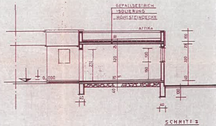
SCHNITT 2
