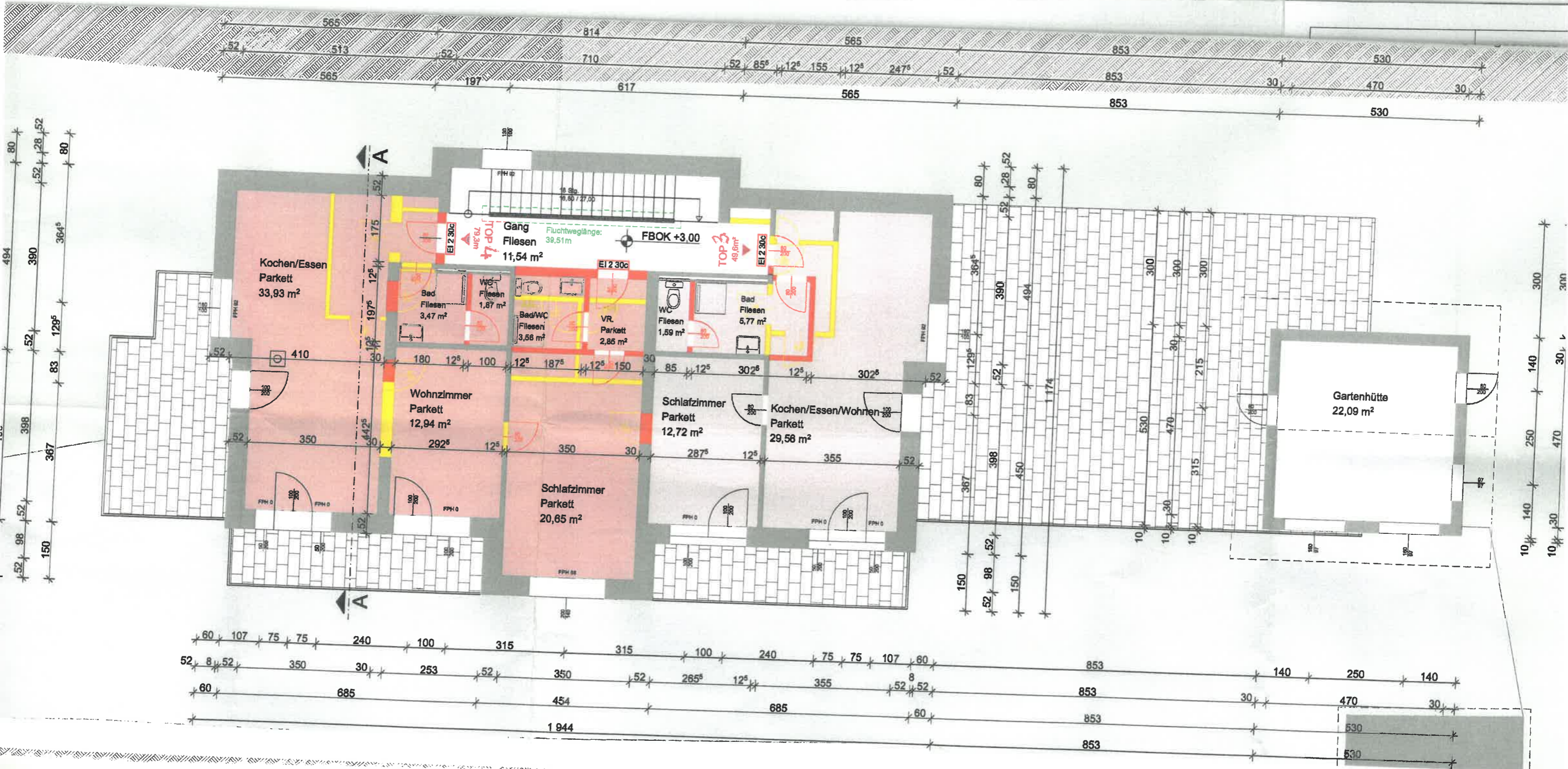
Erdgeschoss 1
