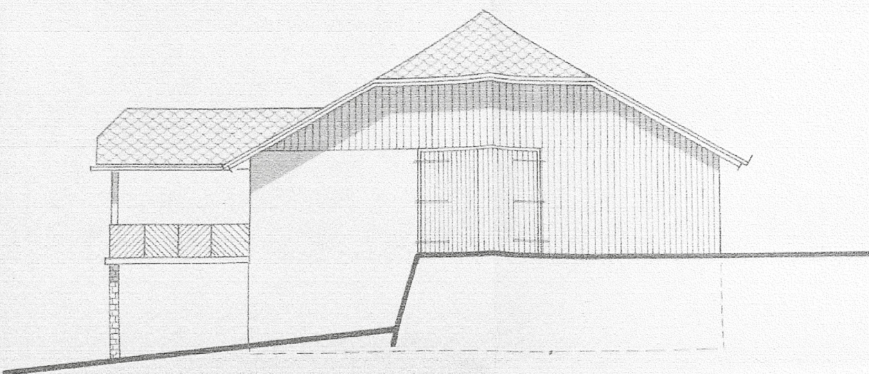
WESTANSICHT
