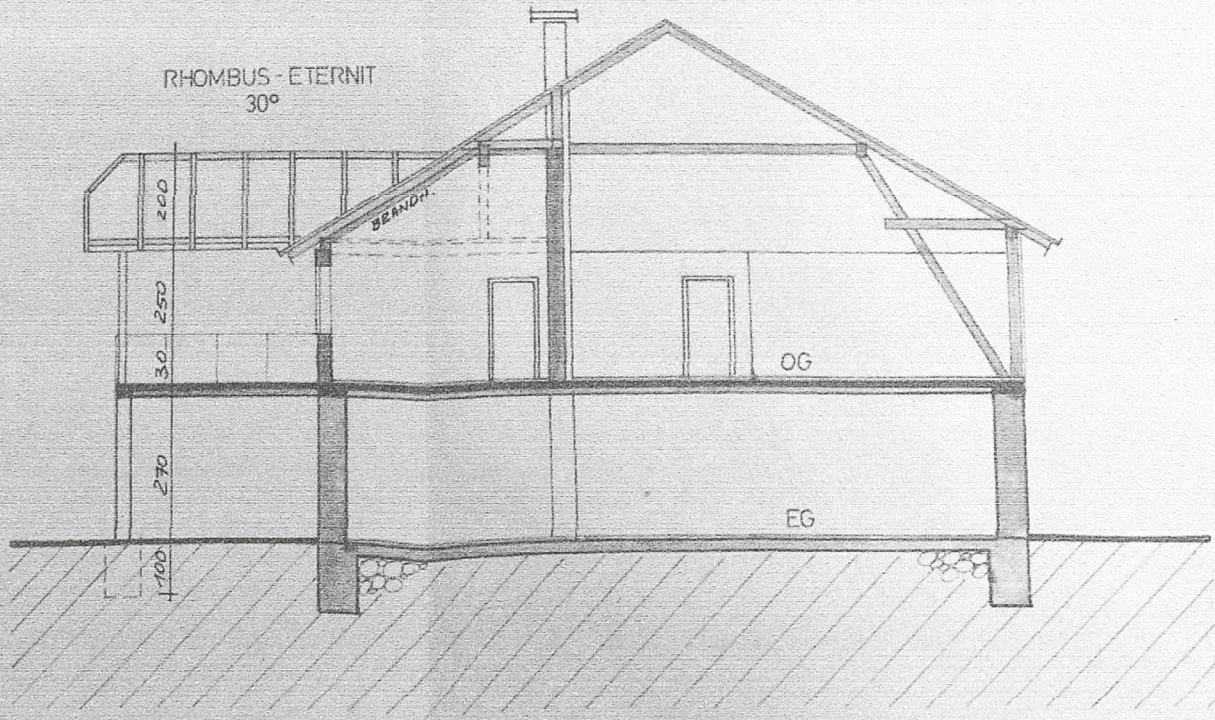
SCHNITT AA
