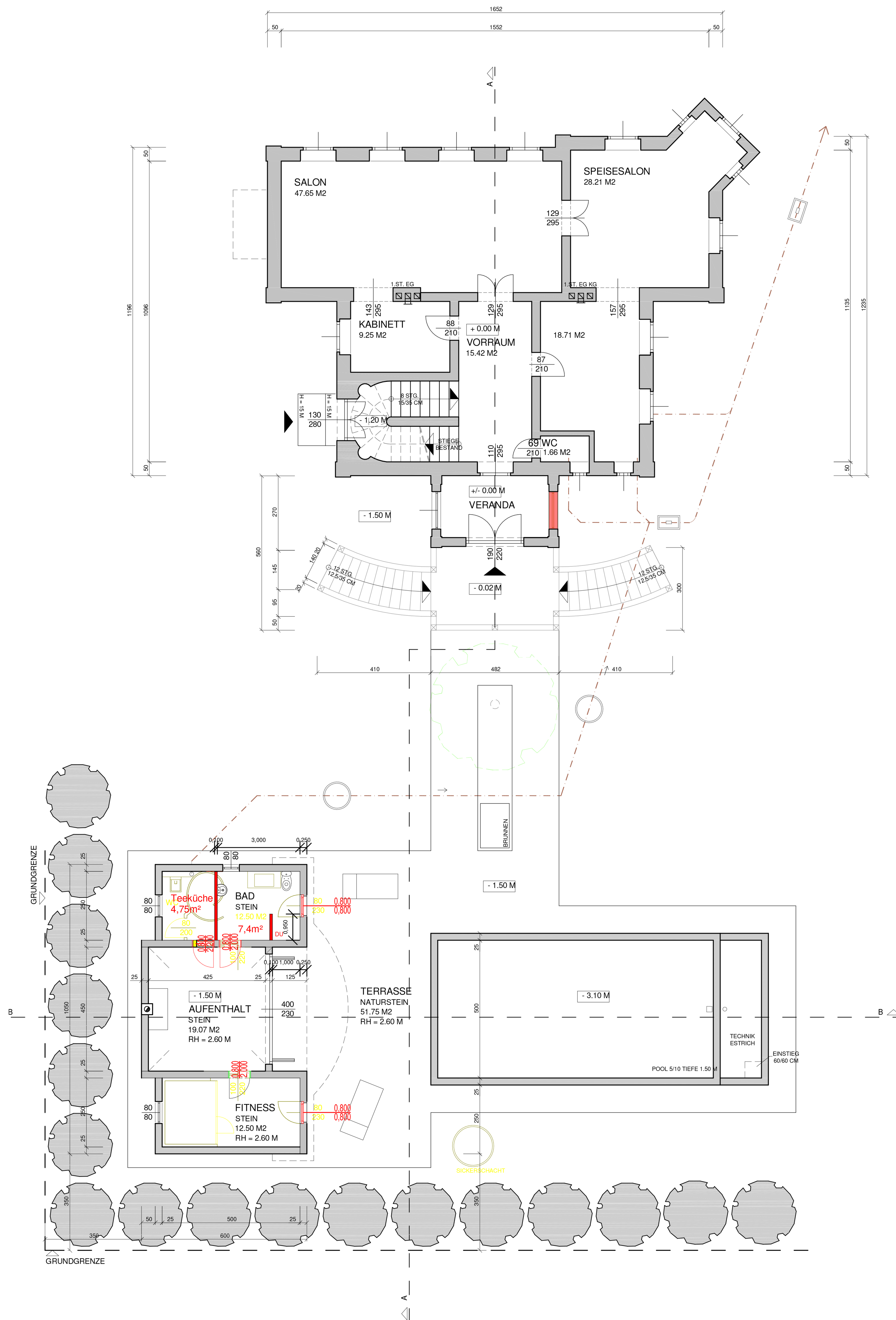
ERDGESCHOSS M 1:100
