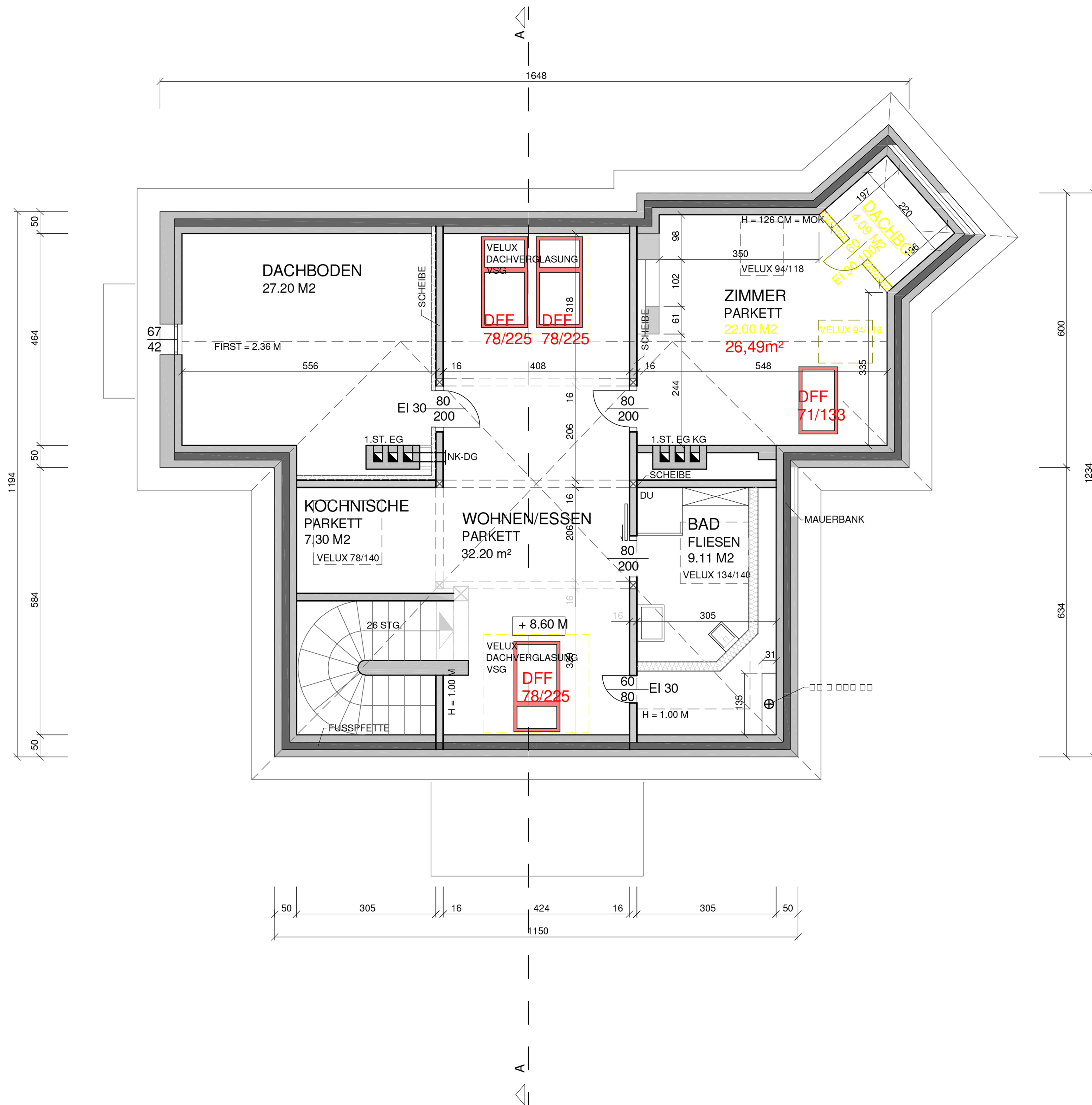
DACHGESCHOSS M 1:100
