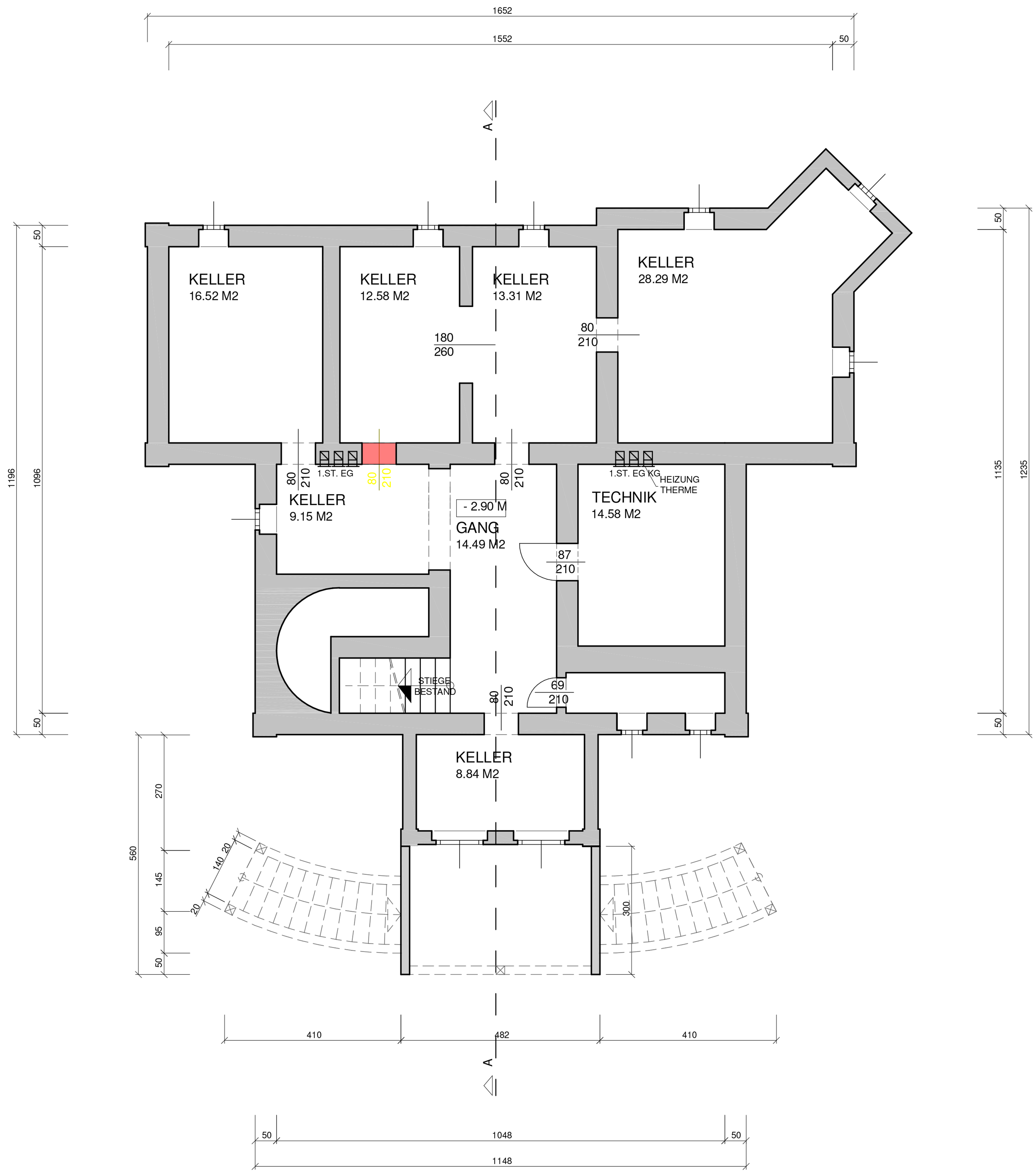
KELLERGESCHOSS M 1:100
